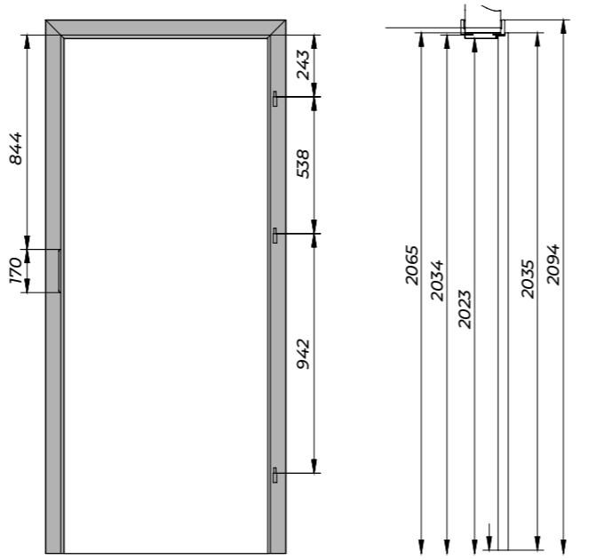
Ościeżnica panelowa OR
