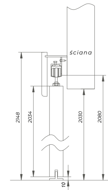
system przesuwnej naściennych bez zabudowy
