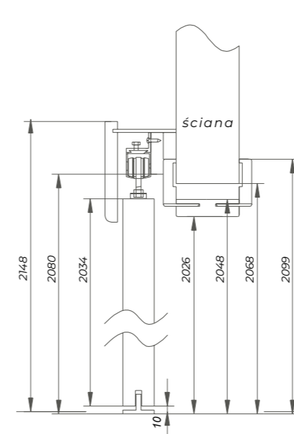
system przesuwnej naściennych z zabudową
