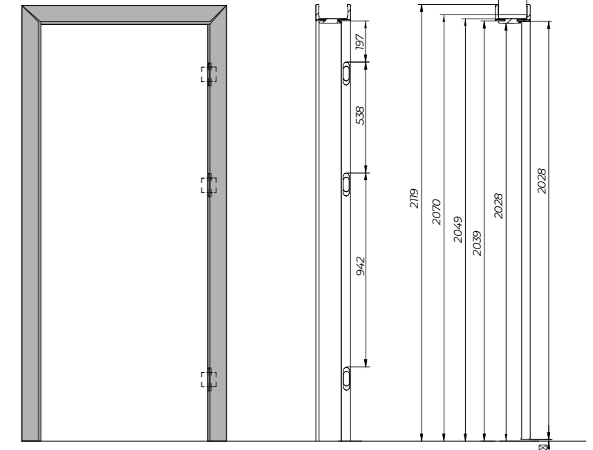
Ościeżnica panelowa OPB
